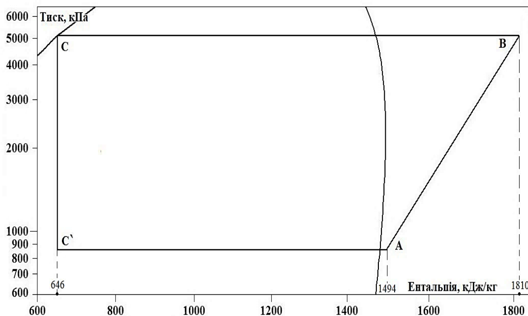
Рис. 5. Цикл ТН з використанням теплоти скидних вод електростанцій: А – вхід до компресора робочого тіла; В – вихід з компресора робочого тіла; С – завершення конденсації робочого тіла
